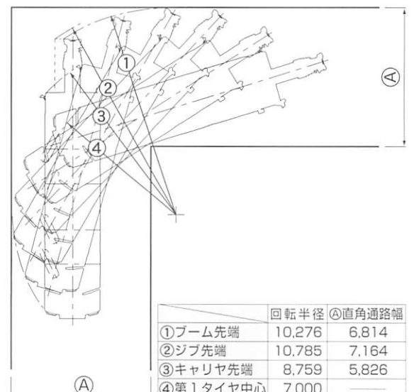
クランプステアリング (8輪)
